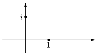
Рис. 1. Вещественные базисные векторы на плоскости комплексных чисел.
