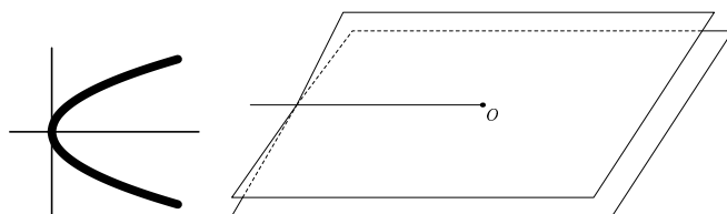
Рис. 15. Группа монодромии функции «квадратный корень» состоит из двух перестановок обоих корней.
