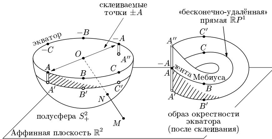
Рис. 9. Построение проективной плоскости приклеиванием ленты Мёбиуса к кругу A'B'C' (или проективной прямой \mathbb{R}P^1 «бесконечно-удалённых» точек к аффинной плоскости \mathbb{R}^2 ).
