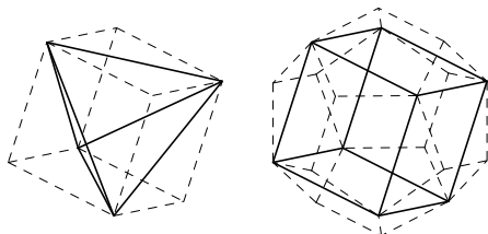
Рис. 11. Тетраэдр, вписанный в куб, и куб, вписанный в додекаэдр.
