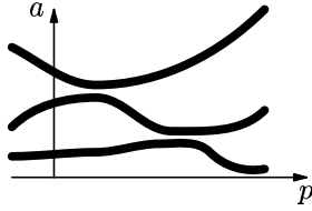
Рис. 18. Расталкивание собственных чисел.
