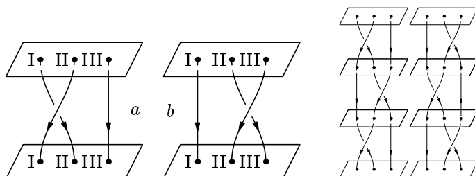
Рис. 19. Косы из трёх нитей на плоскости.
